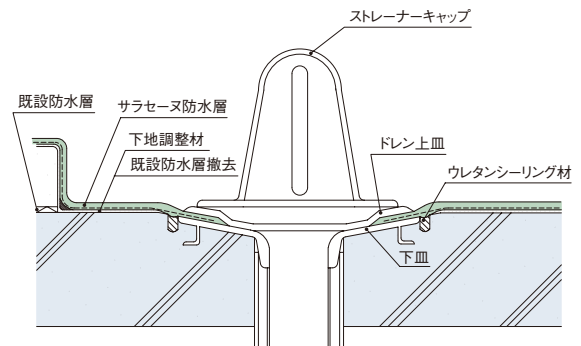
縦引きドレン
