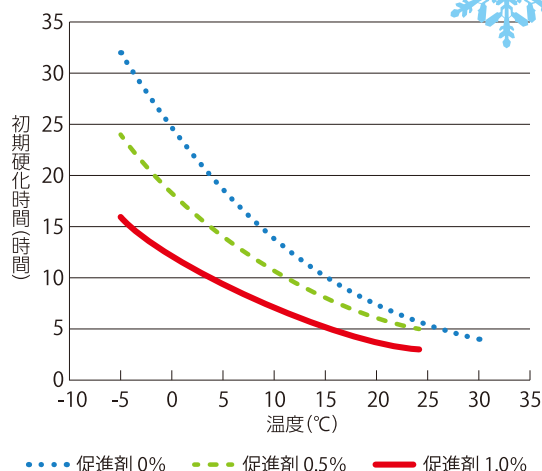
図1 ■サラセーヌEQ硬化性グラフ
