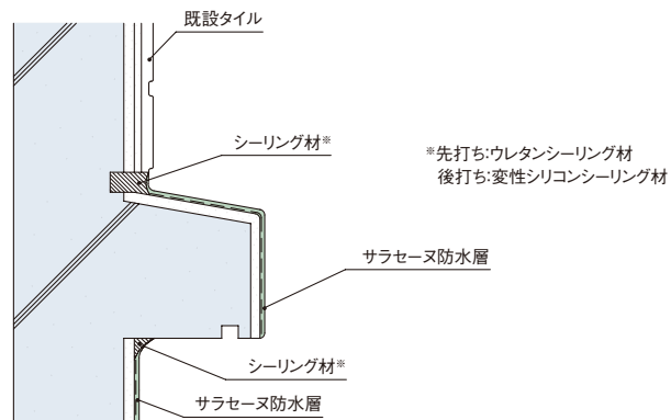
壁面取り合い - 3
