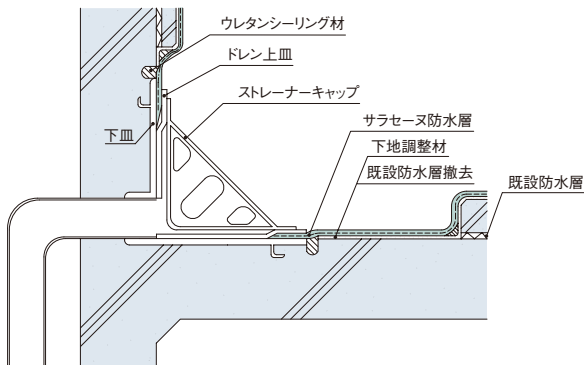
横引きドレン
