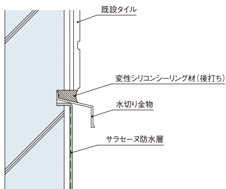
壁面取り合い - 2
