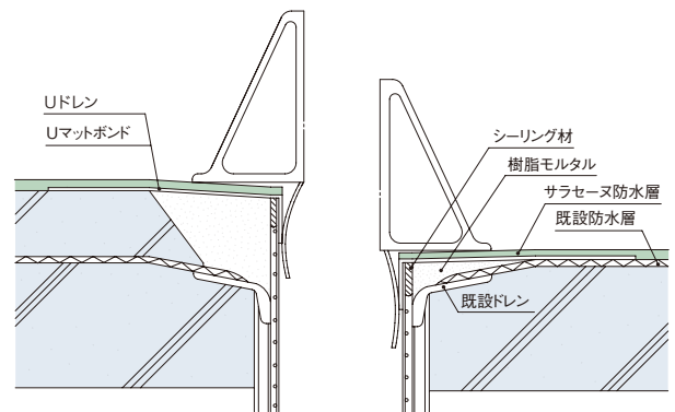
縦引き改修用ドレン「Uドレン タテ」
