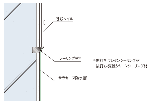
壁面取り合い - 1
