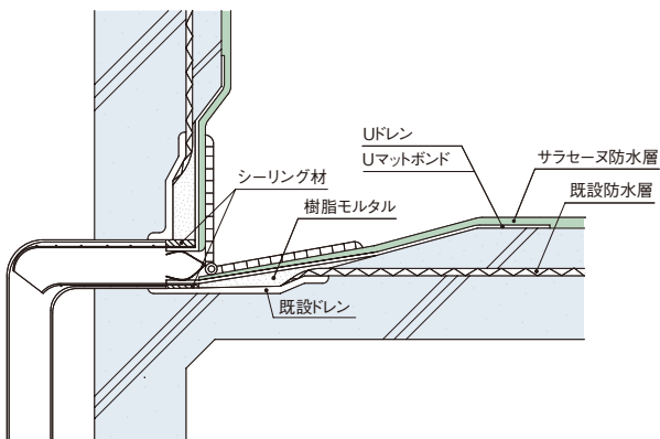
横引き改修用ドレン「Uドレン ヨコ」
