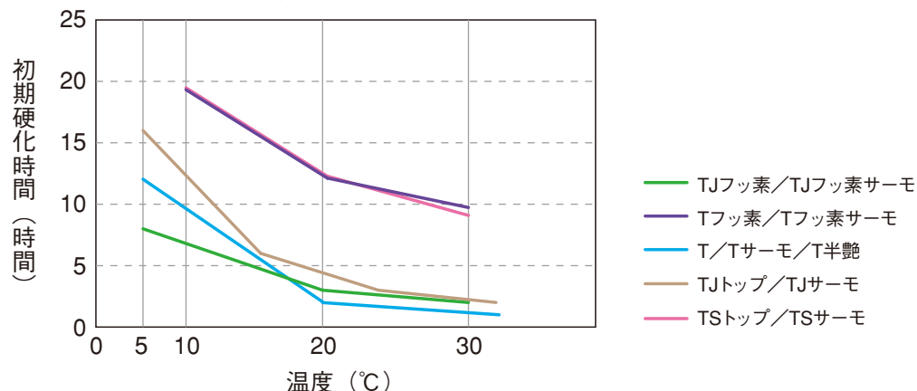
初期硬化時間の目安
